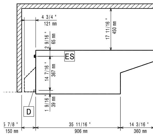
Zij aanzicht
